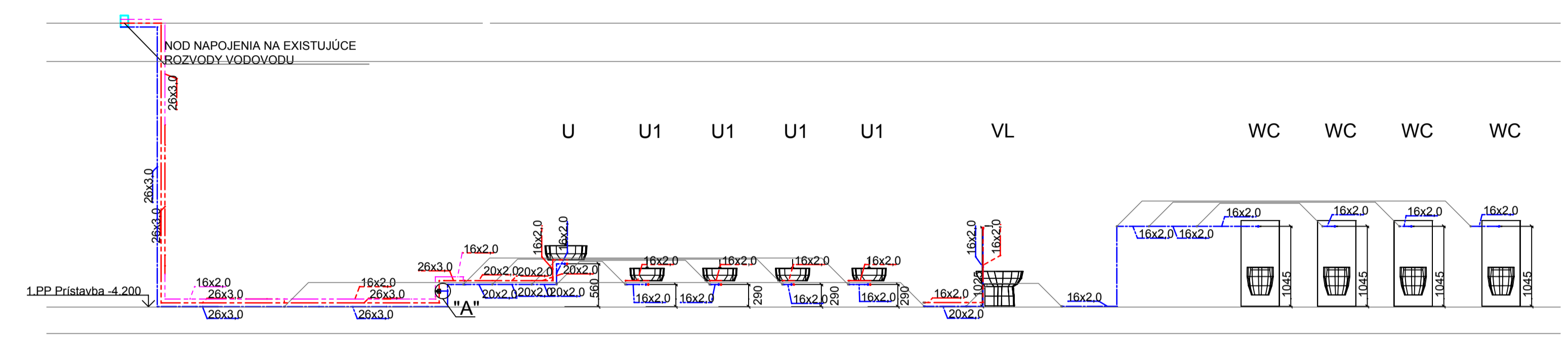
ZVISLÁ SCHÉMA VODOVODU
